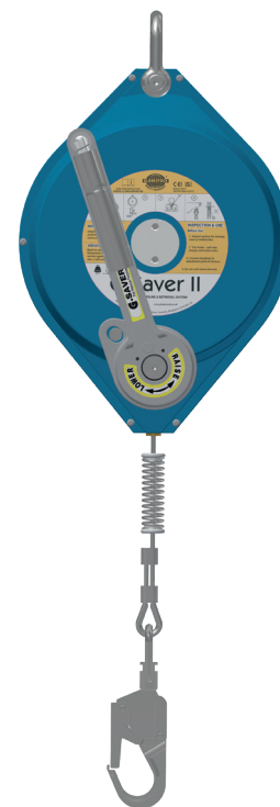
GSE420G / GSE420SSK GSE434G / GSE434SSK 20-34 m
