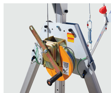
CA284: argano di recupero di emergenza
