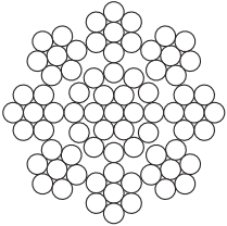
8x7+WS 75 fili/wires
