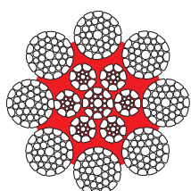
8xK36WS+EPIWRC 407 fili/wires
