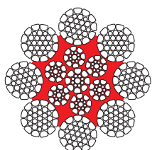
8xK31WS+EPIWRC 367 fili/wires
