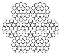
7x19 133 fili/wires
