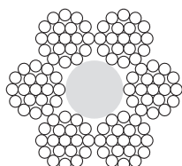
6x19+PP 114 fili/wires
